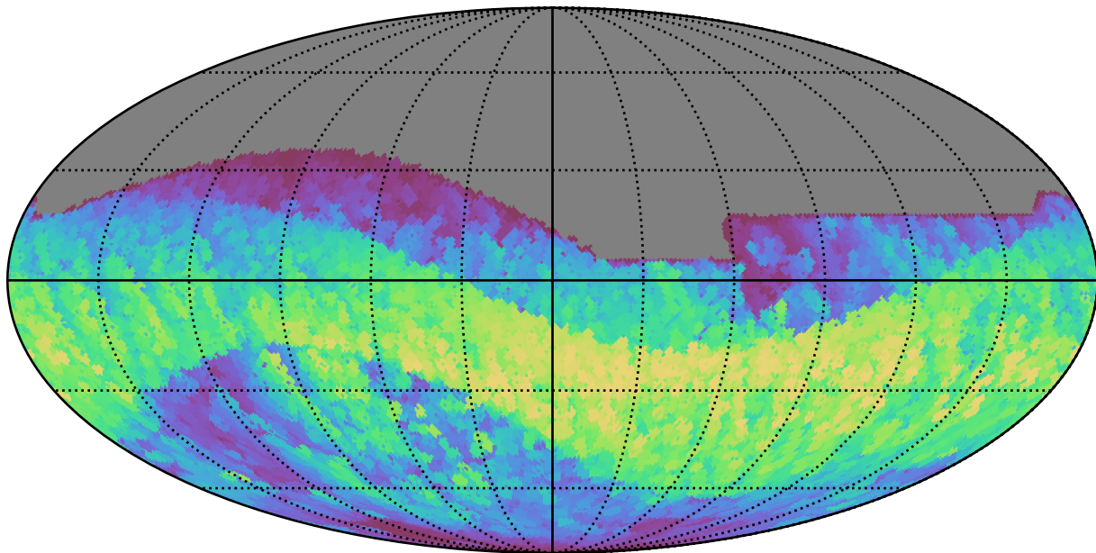
extra_ss_neo3_v3.4_10yrs All sky z band: Max normairmass
