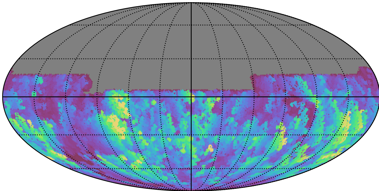
extra_ss_neo3_v3.4_10yrs All sky u band: Max normairmass
