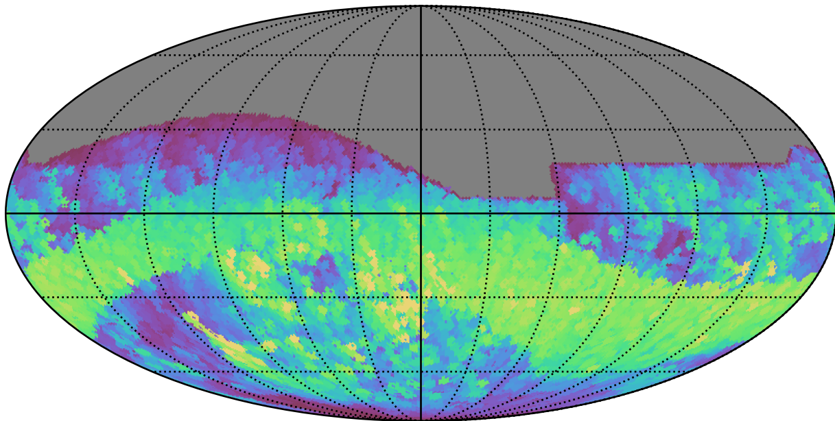
extra_ss_neo3_v3.4_10yrs All sky r band: Max normairmass
