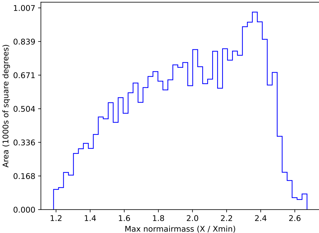
extra_ss_neo3_v3.4_10yrs All sky r band: Max normairmass
