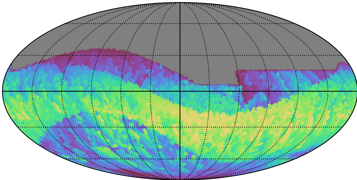
extra_ss_neo3_v3.4_10yrs All sky i band: Max normairmass
