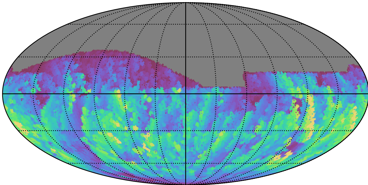
extra_ss_neo3_v3.4_10yrs All sky g band: Max normairmass
