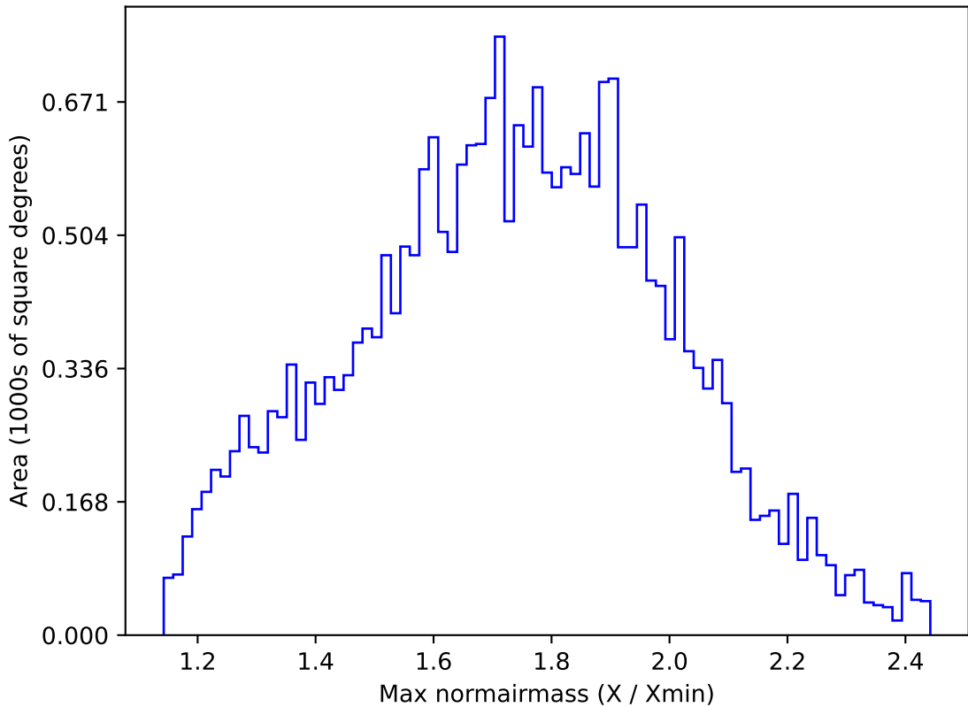
extra_ss_neo3_v3.4_10yrs All sky g band: Max normairmass
