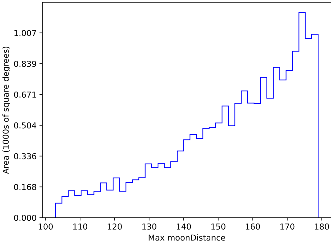
extra_ss_neo3_v3.4_10yrs WFD z band: Max moonDistance
