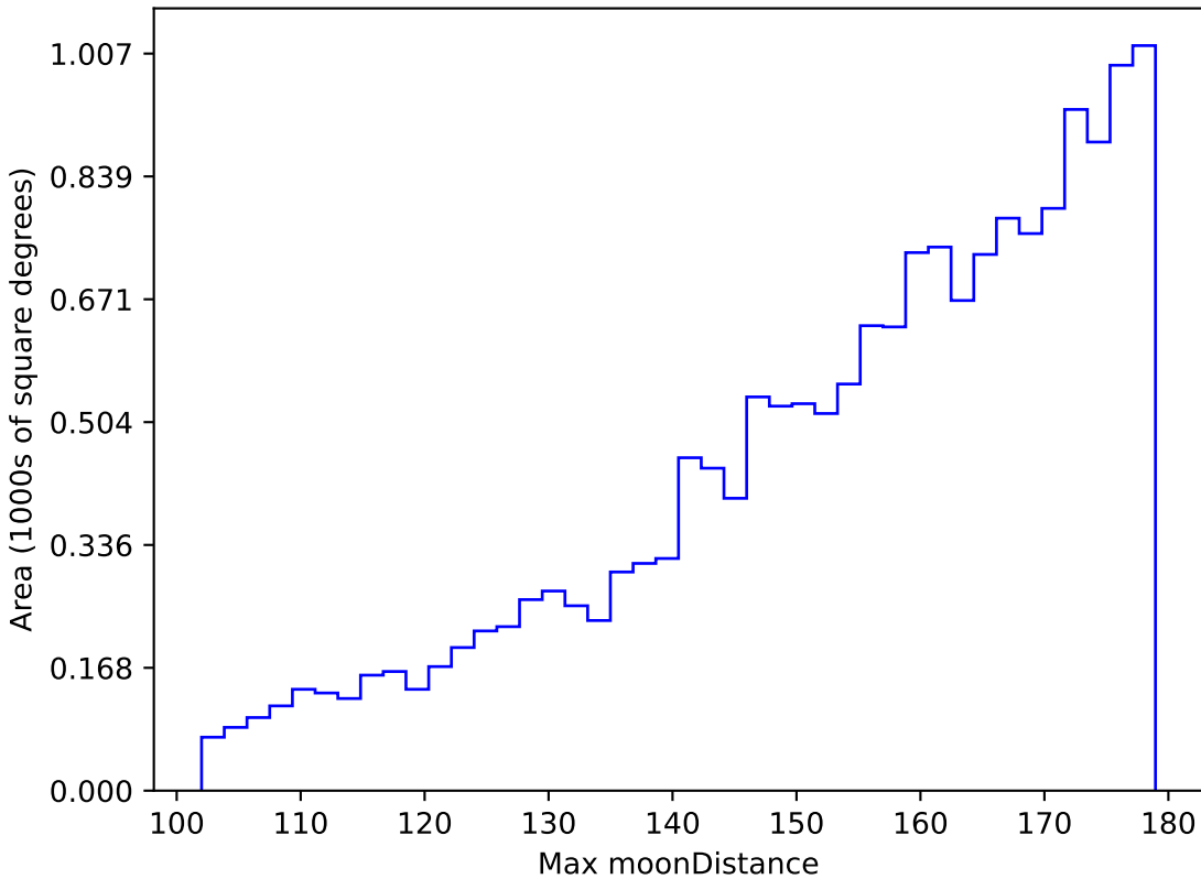
extra_ss_neo3_v3.4_10yrs WFD u band: Max moonDistance
