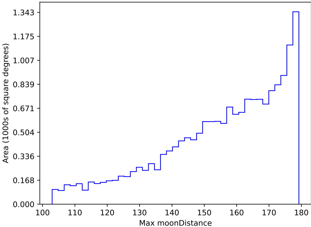
extra_ss_neo3_v3.4_10yrs WFD i band: Max moonDistance
