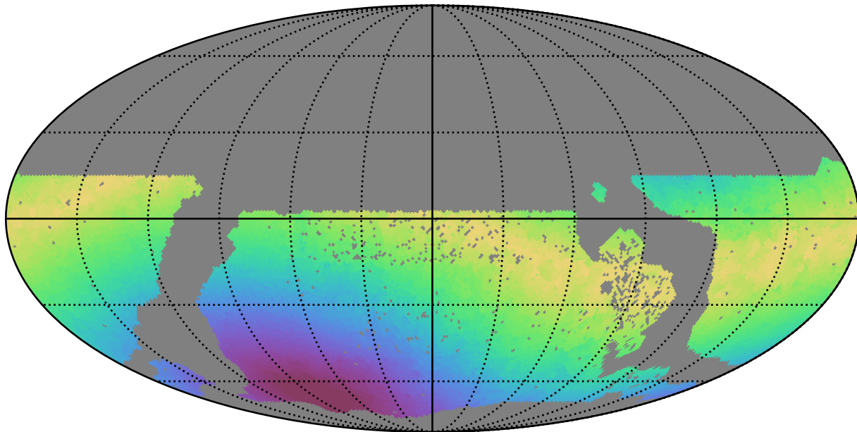
extra_ss_neo3_v3.4_10yrs WFD g band: Max moonDistance
