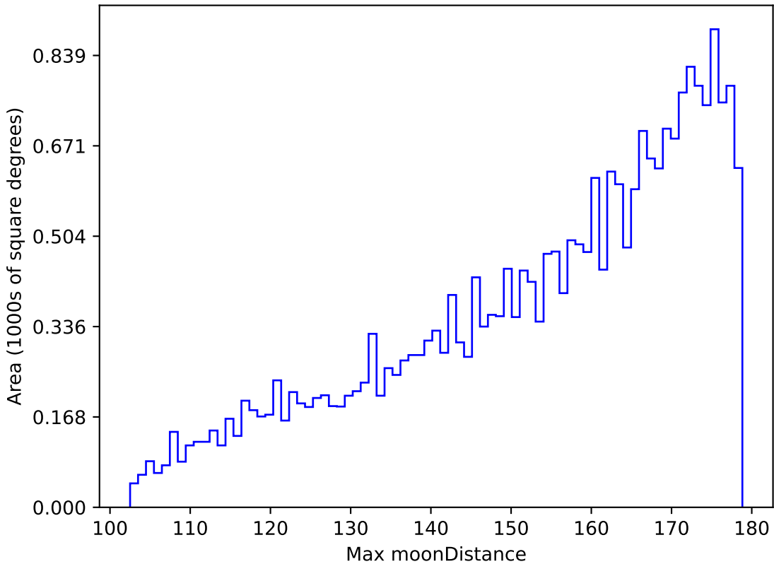
extra_ss_neo3_v3.4_10yrs All sky z band: Max moonDistance
