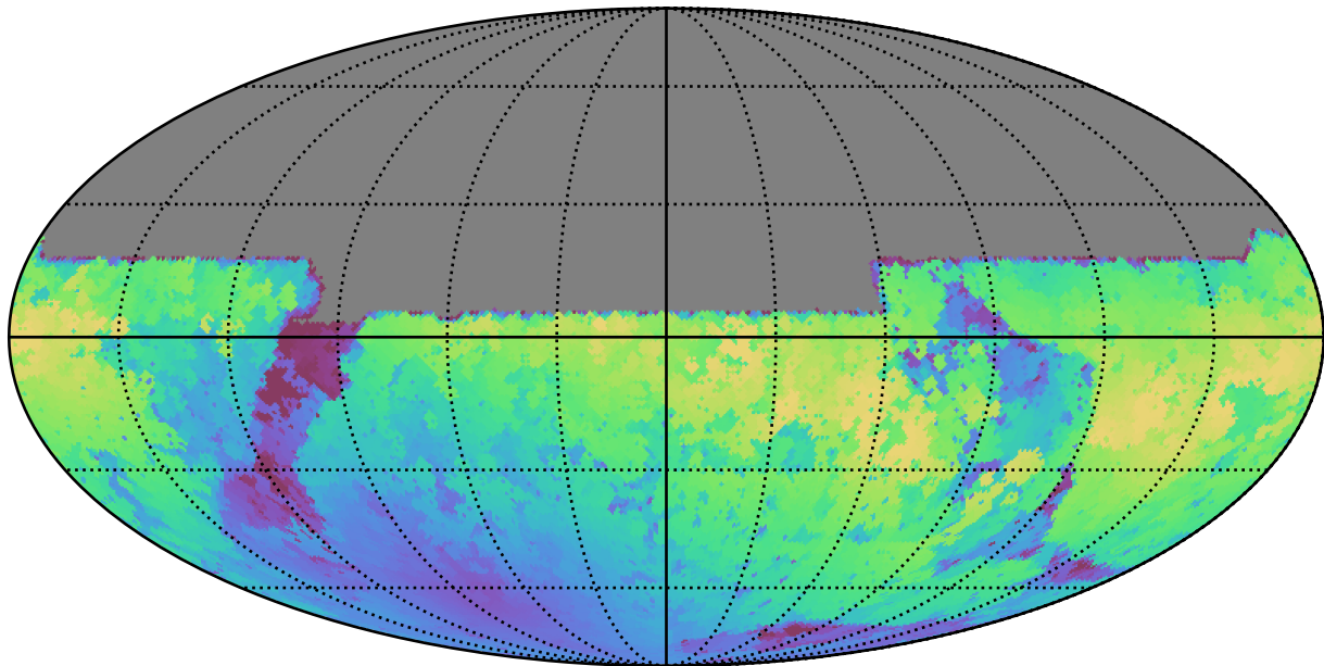
extra_ss_neo3_v3.4_10yrs All sky y band: Max moonDistance
