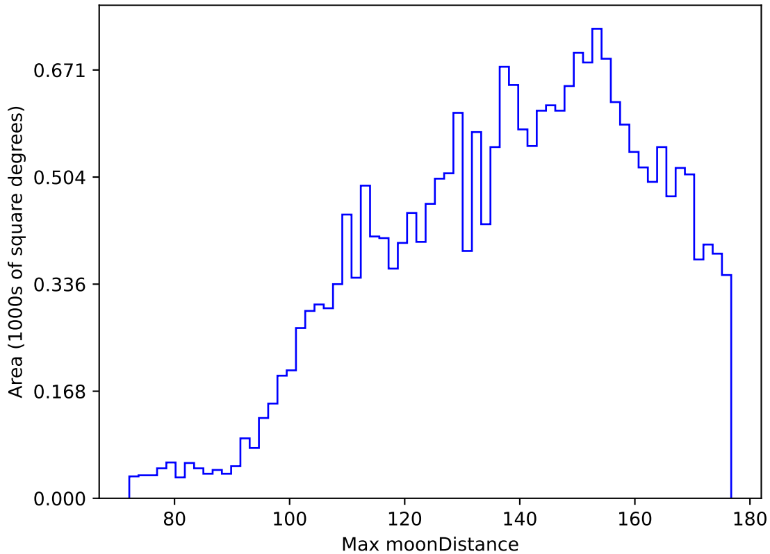
extra_ss_neo3_v3.4_10yrs All sky y band: Max moonDistance
