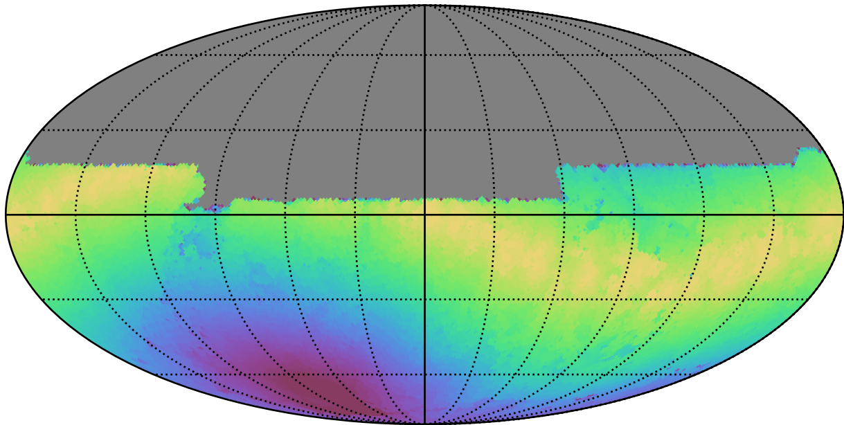
extra_ss_neo3_v3.4_10yrs All sky u band: Max moonDistance
