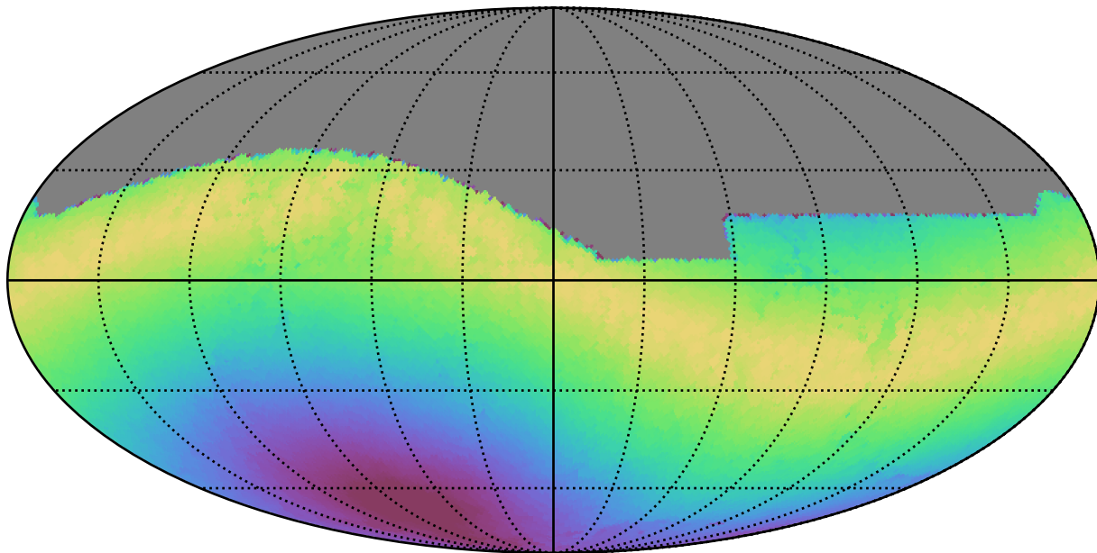
extra_ss_neo3_v3.4_10yrs All sky r band: Max moonDistance
