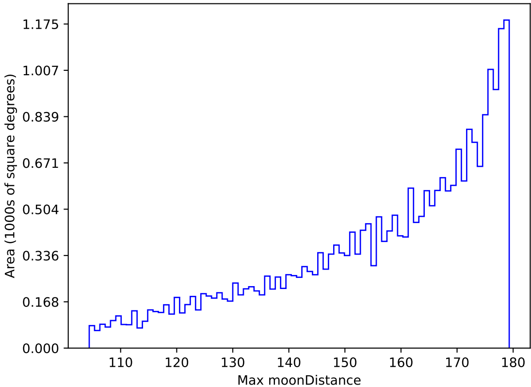
extra_ss_neo3_v3.4_10yrs All sky r band: Max moonDistance
