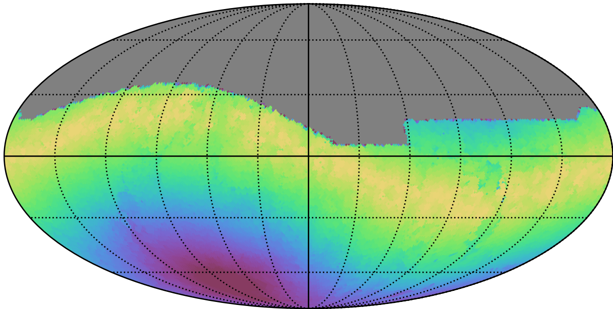
extra_ss_neo3_v3.4_10yrs All sky g band: Max moonDistance
