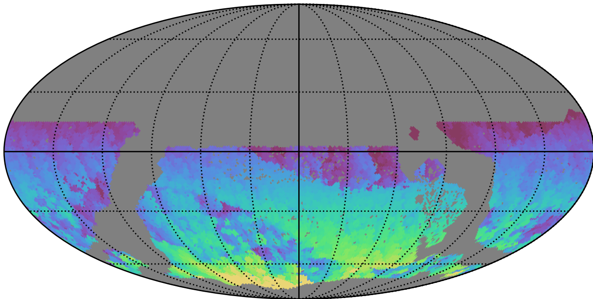
extra_ss_neo3_v3.4_10yrs WFD z band: Max HA
