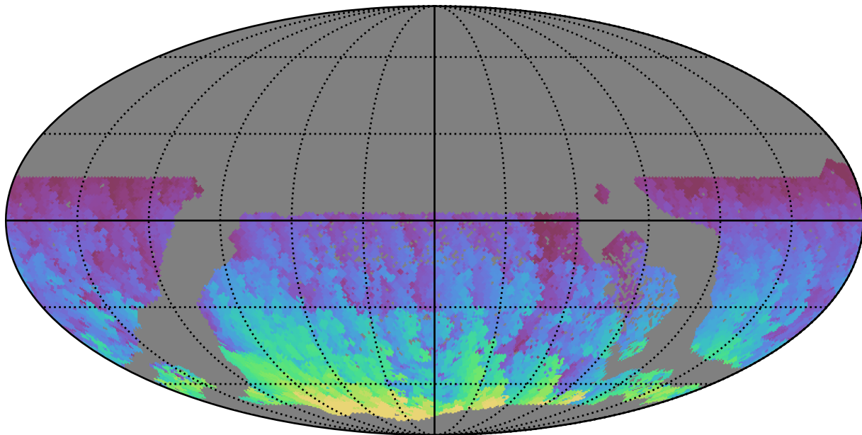
extra_ss_neo3_v3.4_10yrs WFD y band: Max HA
