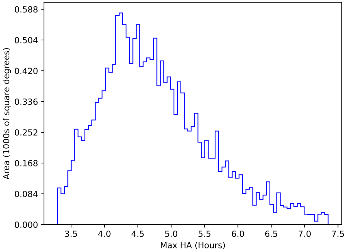
extra_ss_neo3_v3.4_10yrs WFD y band: Max HA
