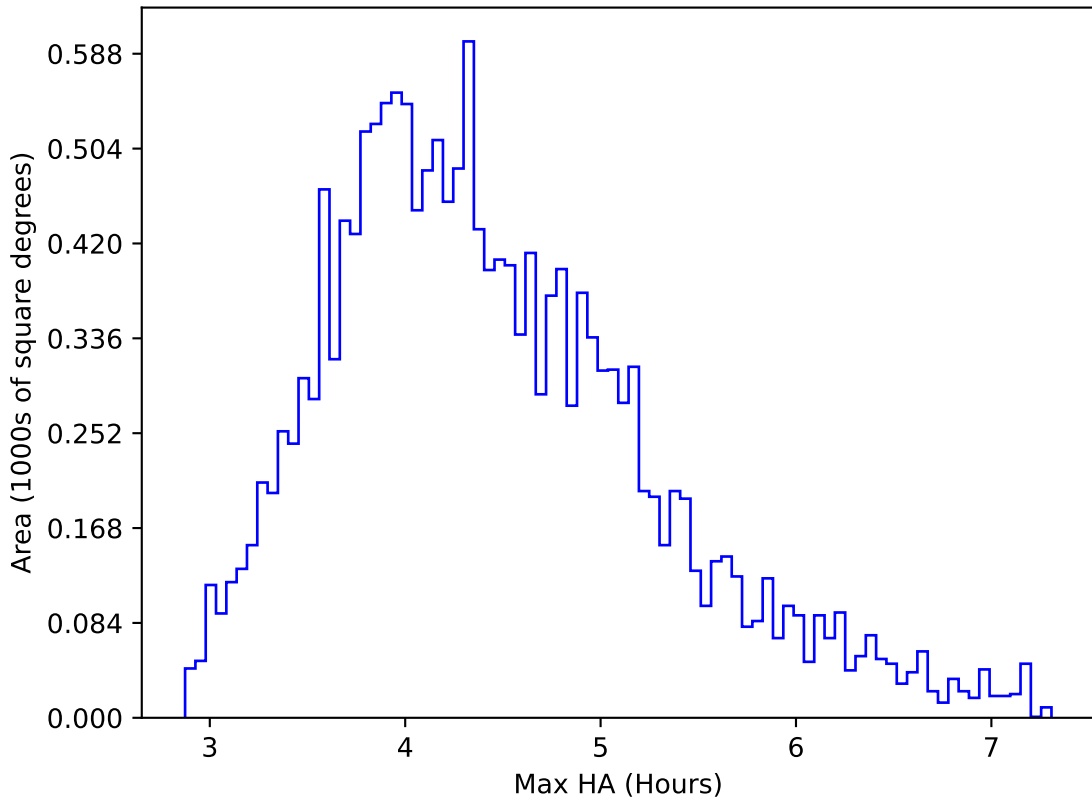
extra_ss_neo3_v3.4_10yrs WFD r band: Max HA
