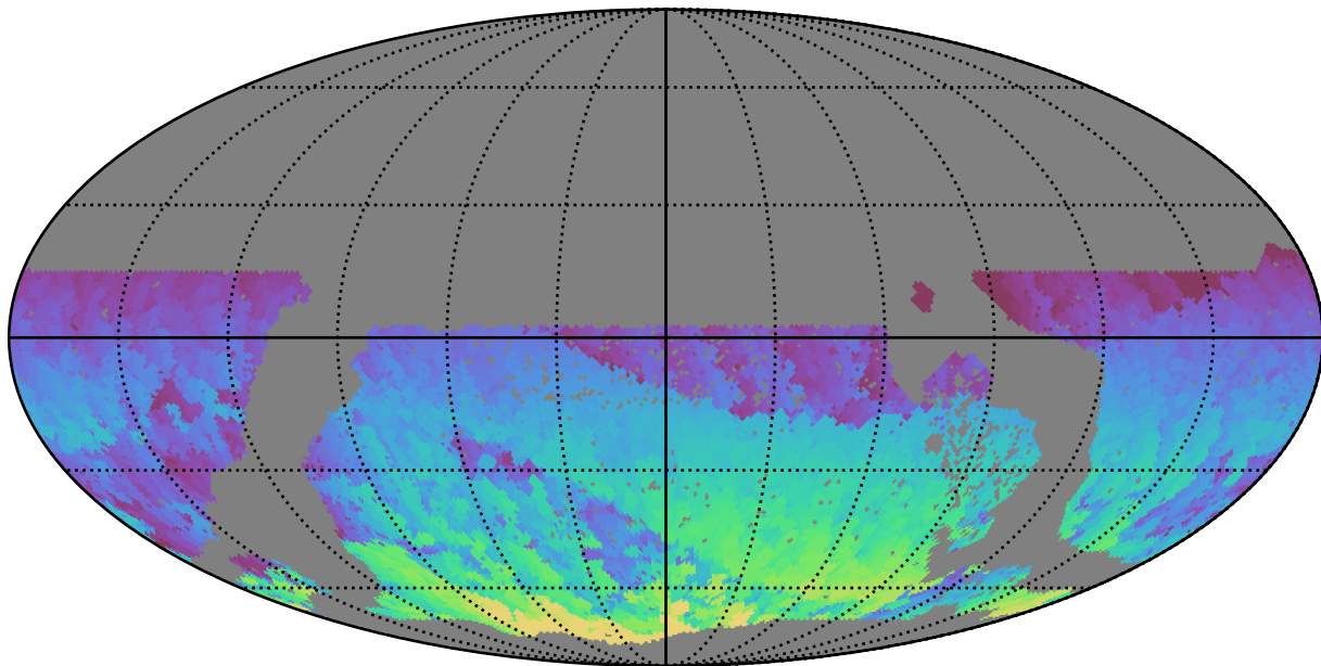
extra_ss_neo3_v3.4_10yrs WFD i band: Max HA
