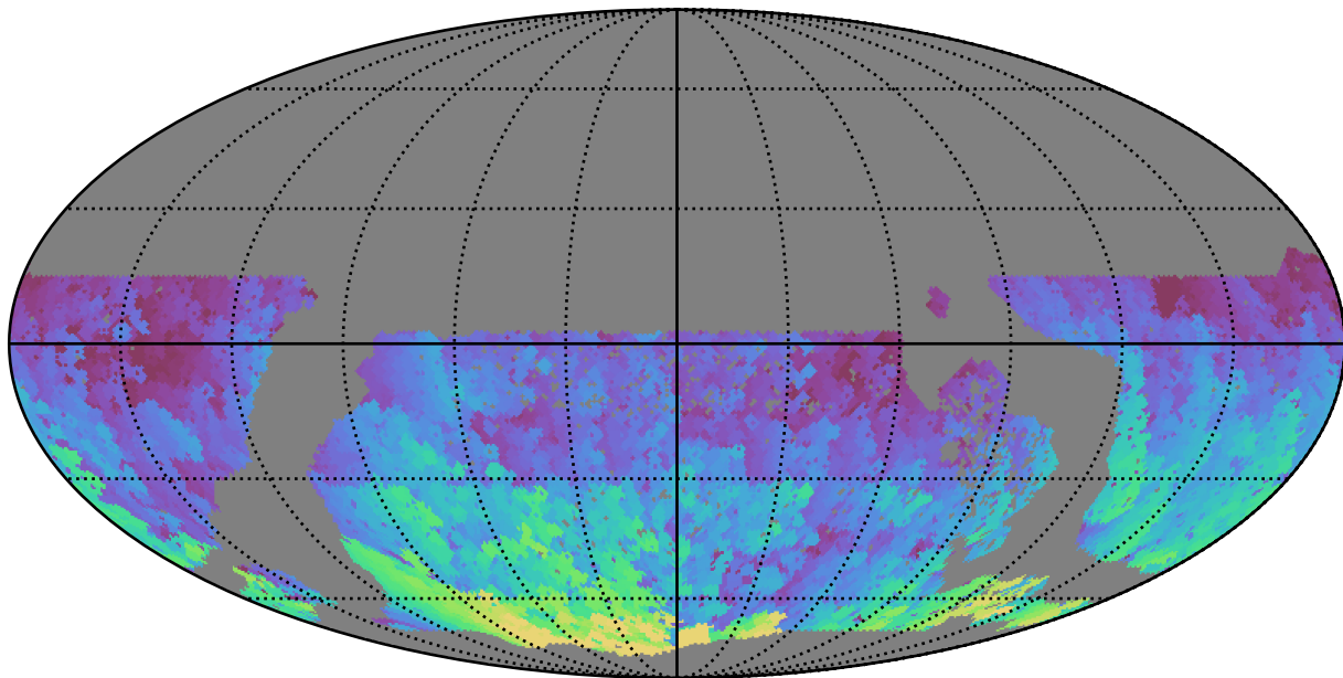
extra_ss_neo3_v3.4_10yrs WFD g band: Max HA
