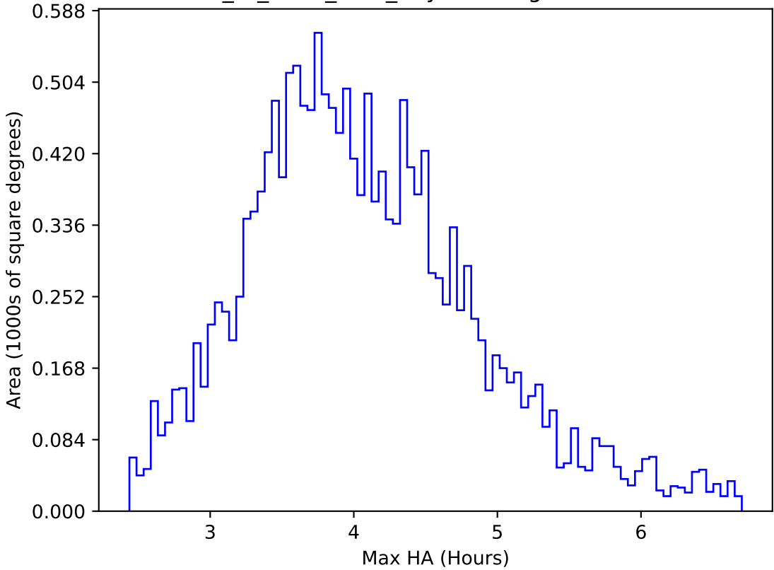
extra_ss_neo3_v3.4_10yrs WFD g band: Max HA
