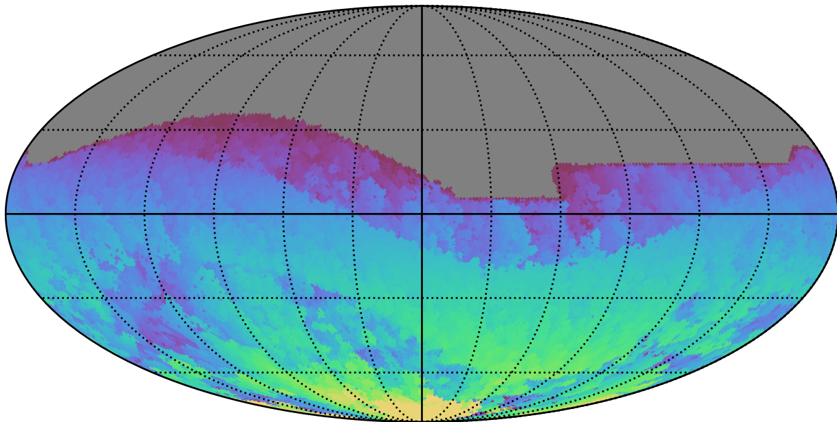
extra_ss_neo3_v3.4_10yrs All sky z band: Max HA
