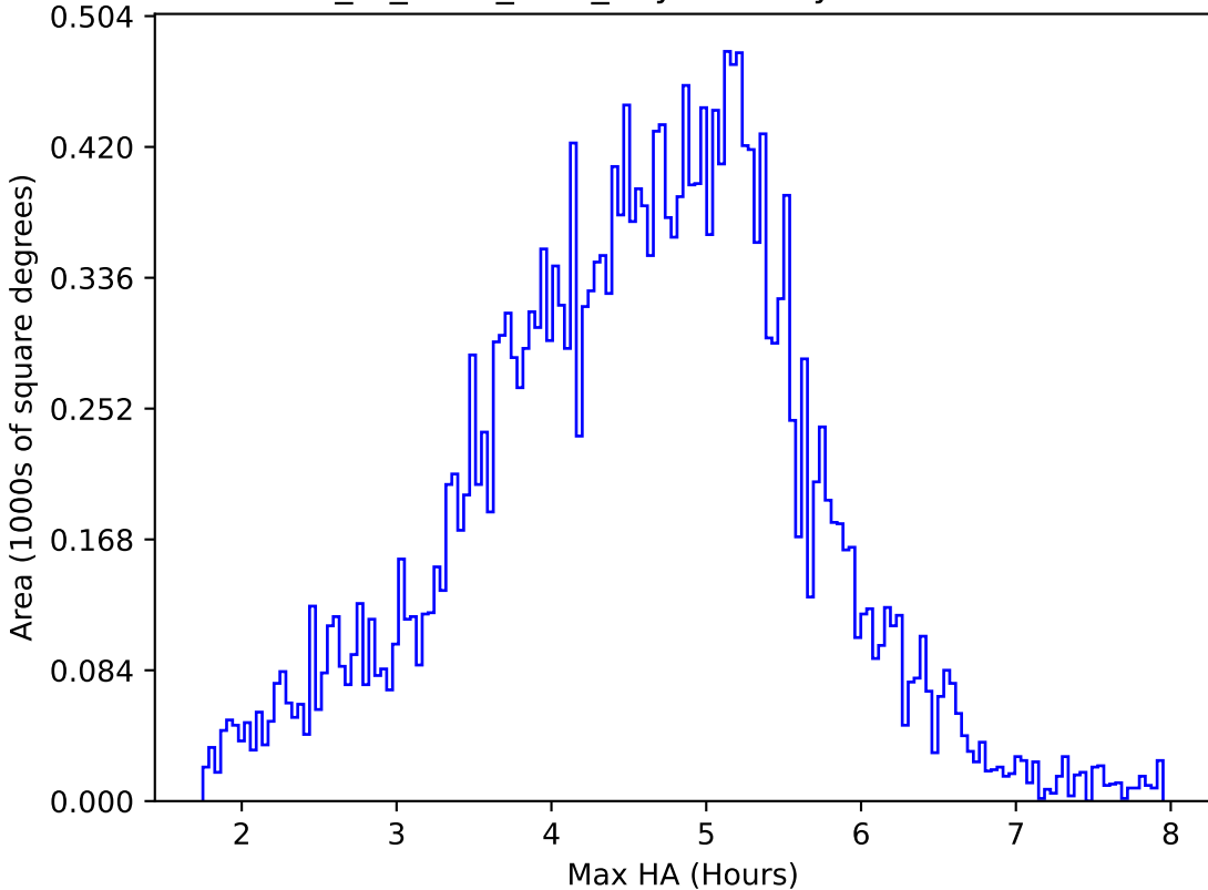
extra_ss_neo3_v3.4_10yrs All sky z band: Max HA
