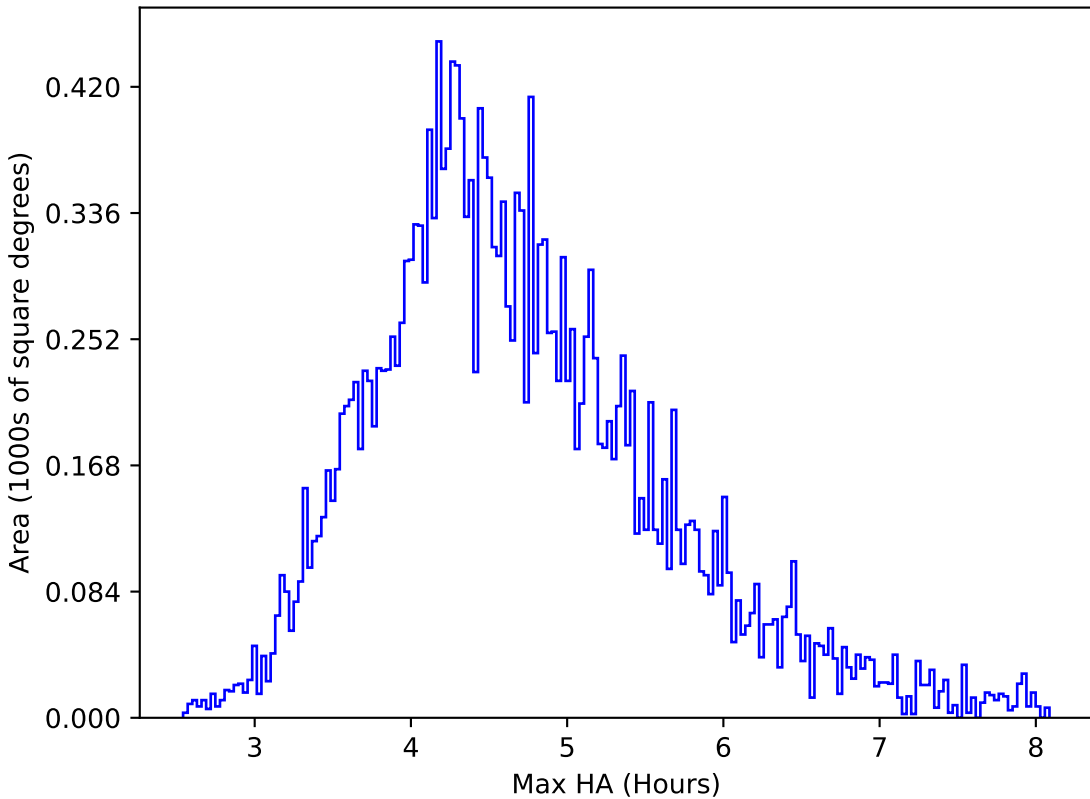
extra_ss_neo3_v3.4_10yrs All sky y band: Max HA
