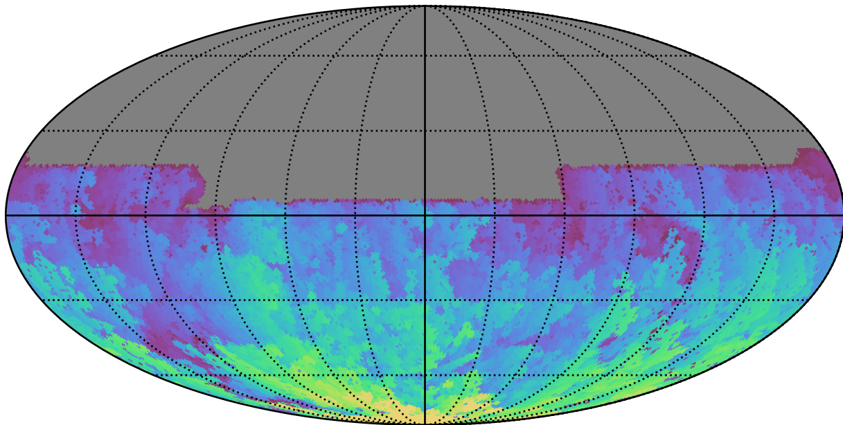
extra_ss_neo3_v3.4_10yrs All sky u band: Max HA
