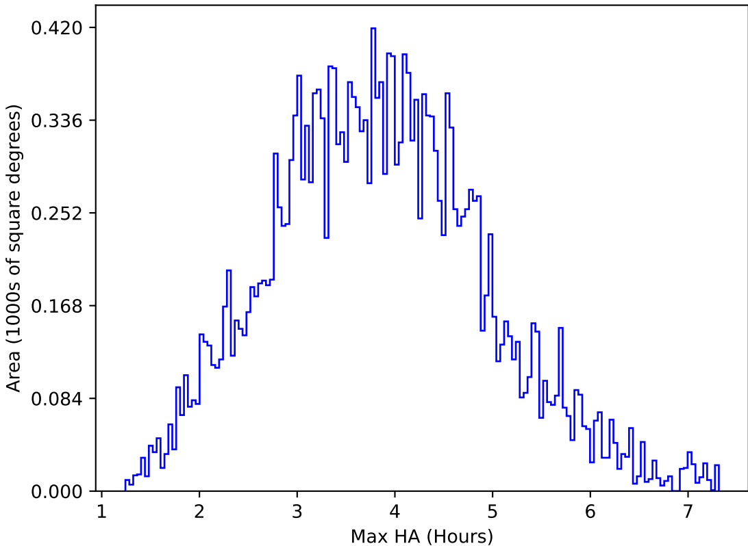
extra_ss_neo3_v3.4_10yrs All sky u band: Max HA
