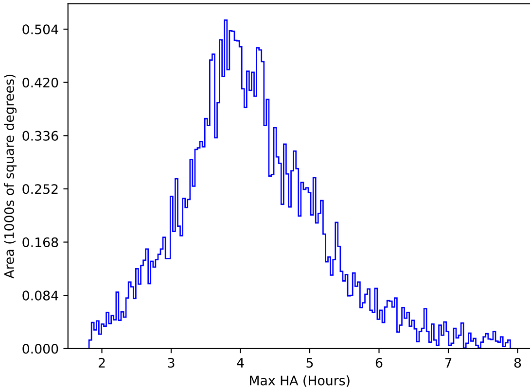
extra_ss_neo3_v3.4_10yrs All sky r band: Max HA
