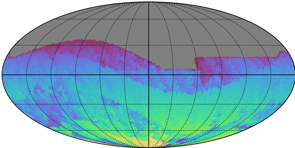
extra_ss_neo3_v3.4_10yrs All sky i band: Max HA
