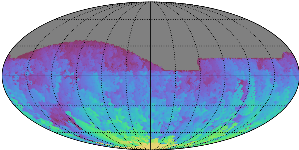
extra_ss_neo3_v3.4_10yrs All sky g band: Max HA
