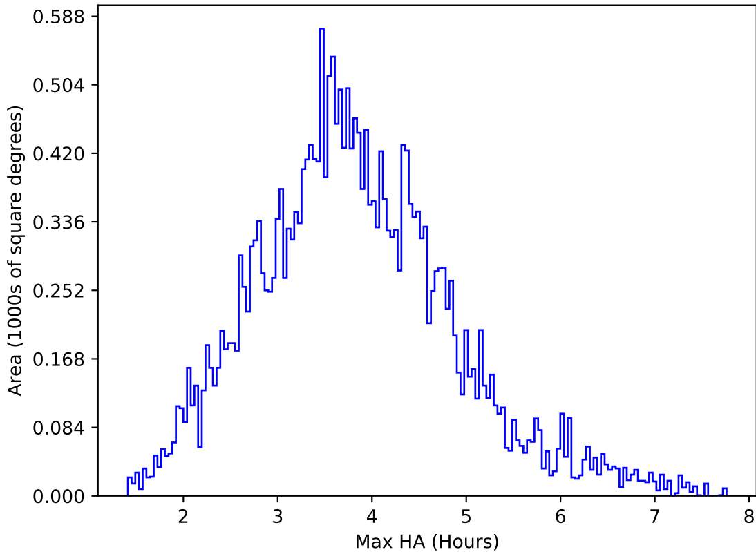
extra_ss_neo3_v3.4_10yrs All sky g band: Max HA
