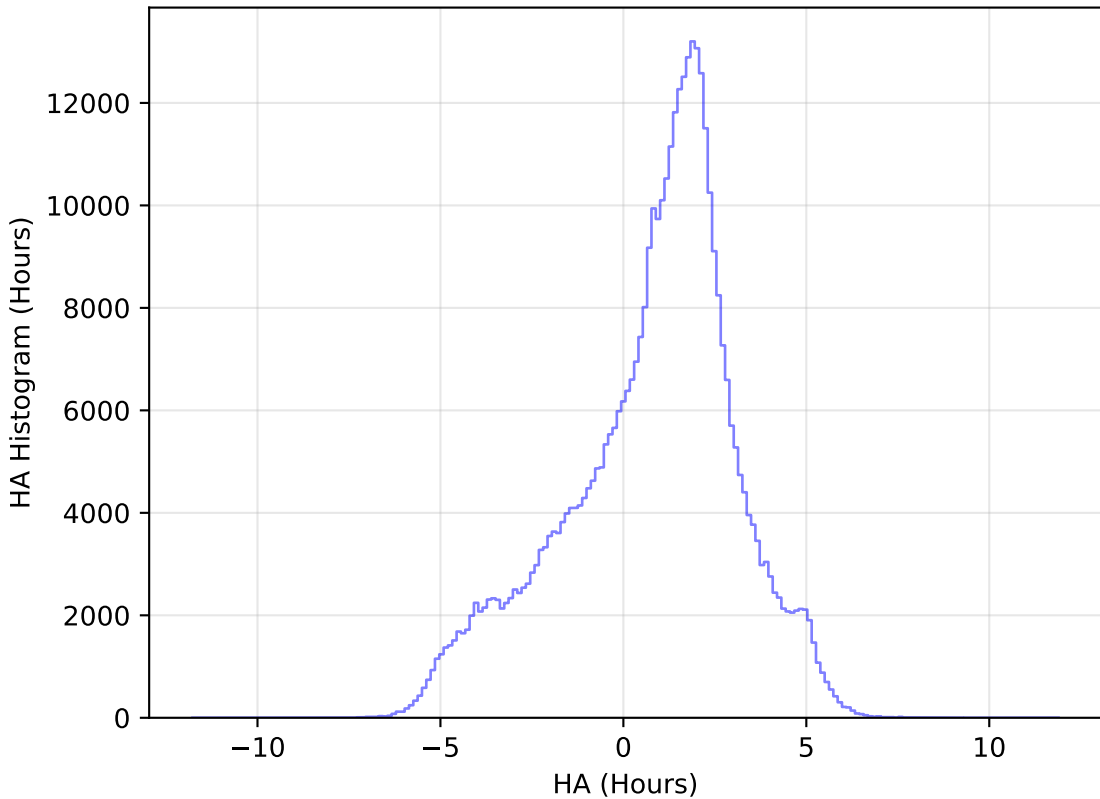
extra_ss_neo3_v3.4_10yrs All sky z band: HA Histogram
