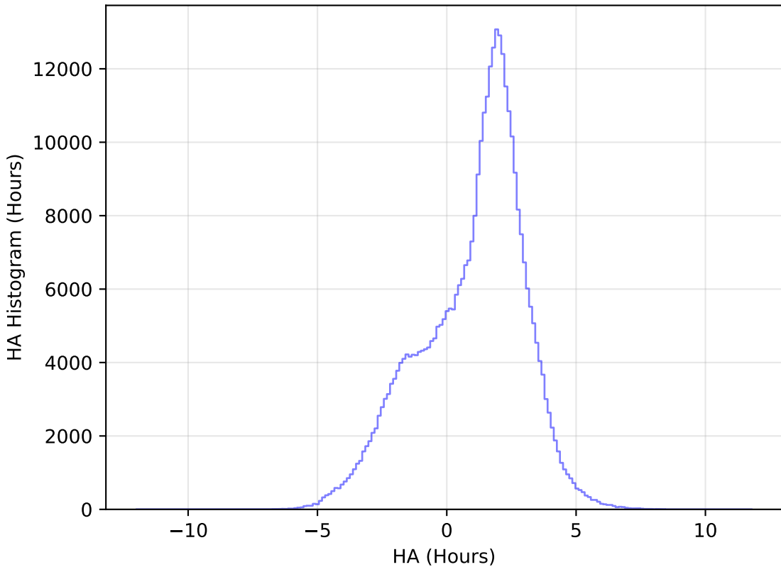
extra_ss_neo3_v3.4_10yrs All sky y band: HA Histogram
