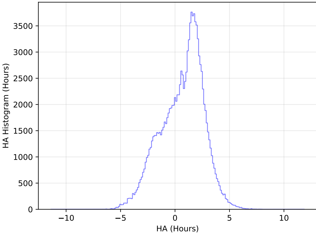
extra_ss_neo3_v3.4_10yrs All sky u band: HA Histogram
