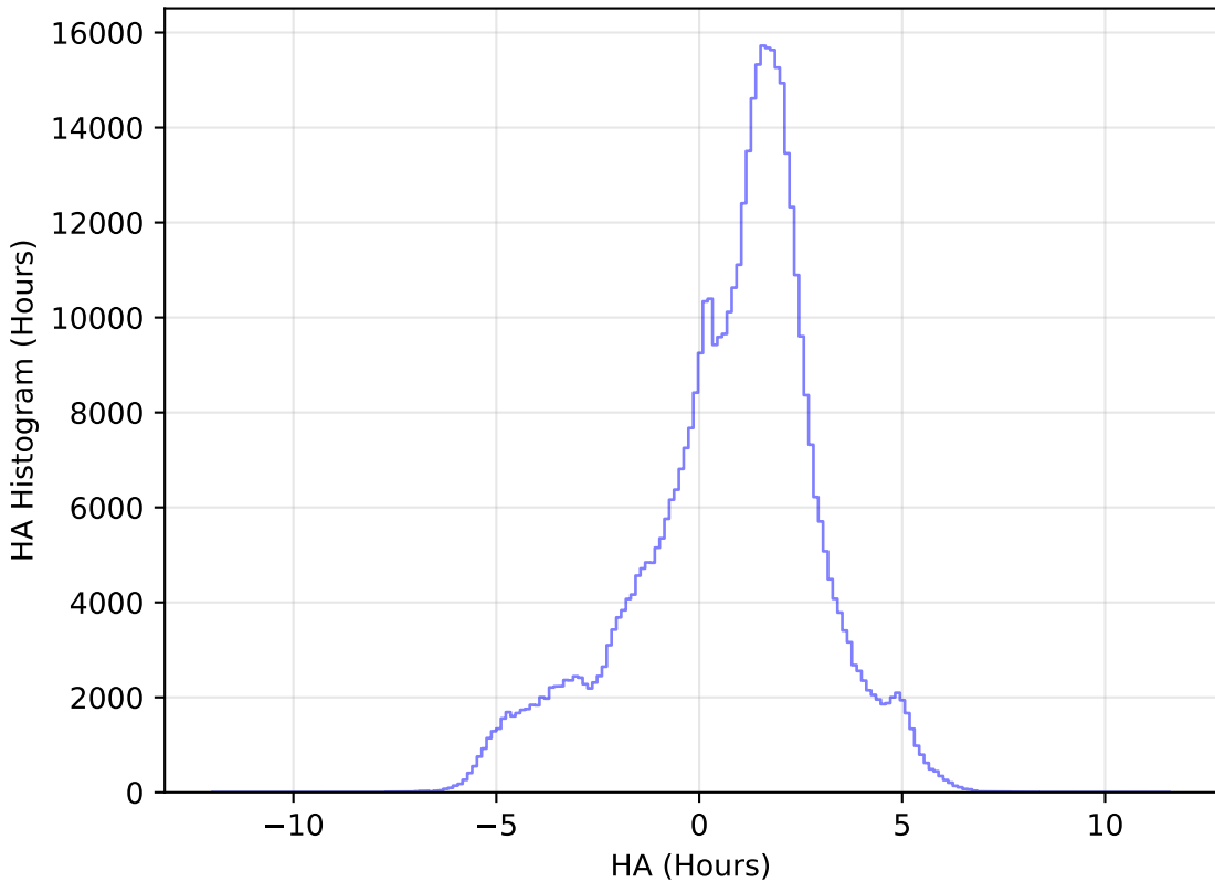
extra_ss_neo3_v3.4_10yrs All sky i band: HA Histogram
