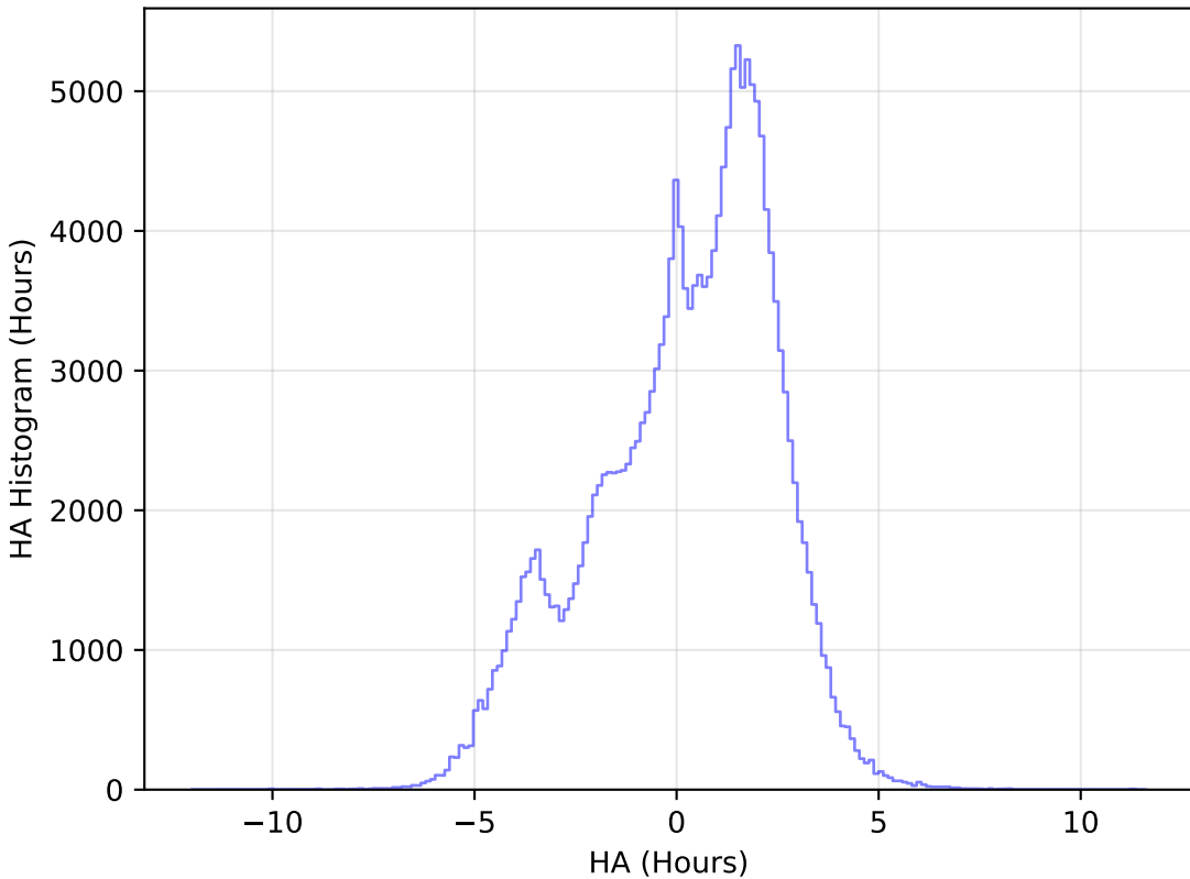
extra_ss_neo3_v3.4_10yrs All sky g band: HA Histogram
