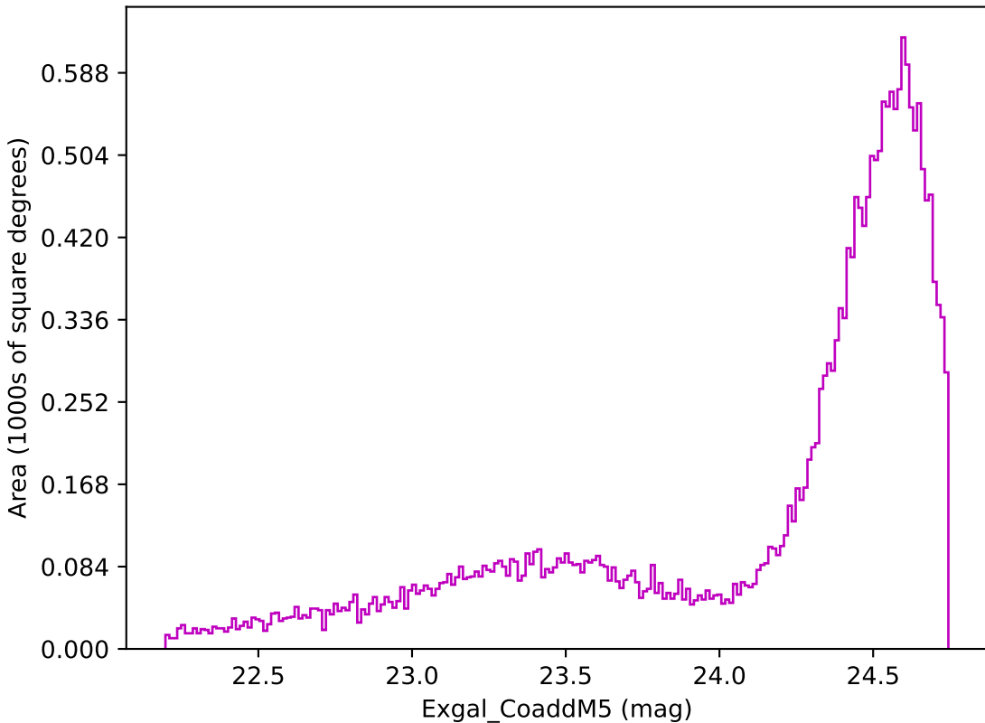
extra_ss_neo3_v3.4_10yrs Yr 1 z band: Exgal_CoaddM5
