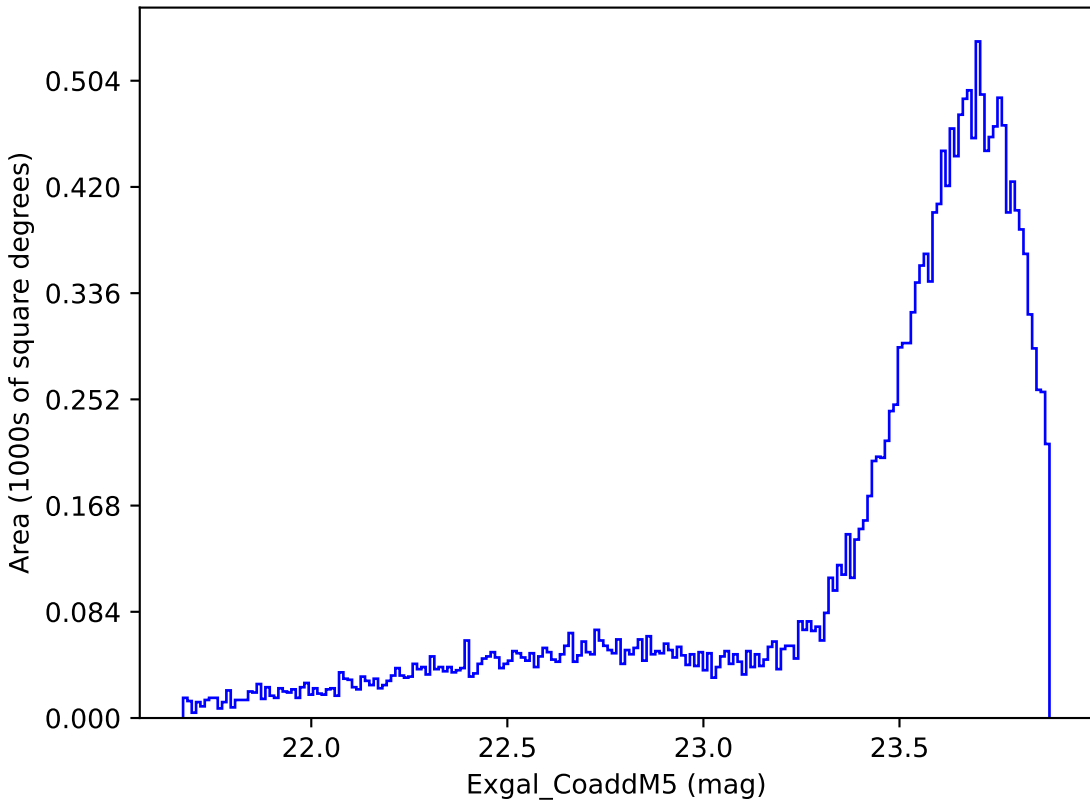
extra_ss_neo3_v3.4_10yrs Yr 1 y band: Exgal_CoaddM5
