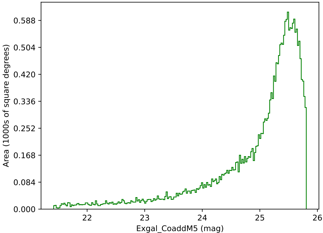
extra_ss_neo3_v3.4_10yrs Yr 1 g band: Exgal_CoaddM5
