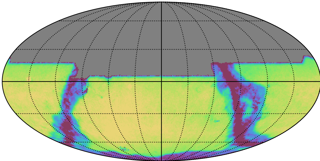
extra_ss_neo3_v3.4_10yrs All sky y band: Exgal_CoaddM5
