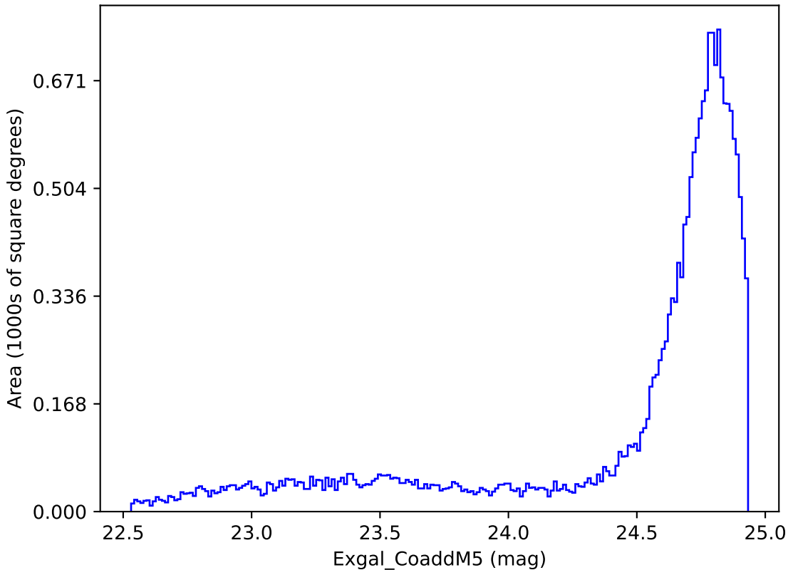
extra_ss_neo3_v3.4_10yrs All sky y band: Exgal_CoaddM5
