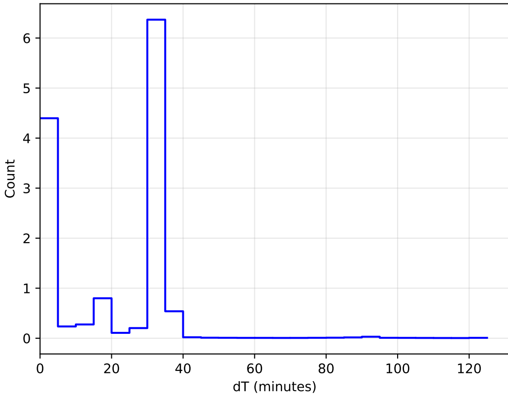
1e6 extra_ss_neo3_v3.4_10yrs All sky: DeltaT Histogram
