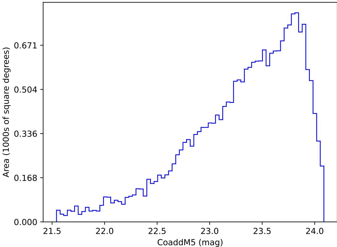
extra_ss_neo3_v3.4_10yrs Yr 3-4 y band: CoaddM5
