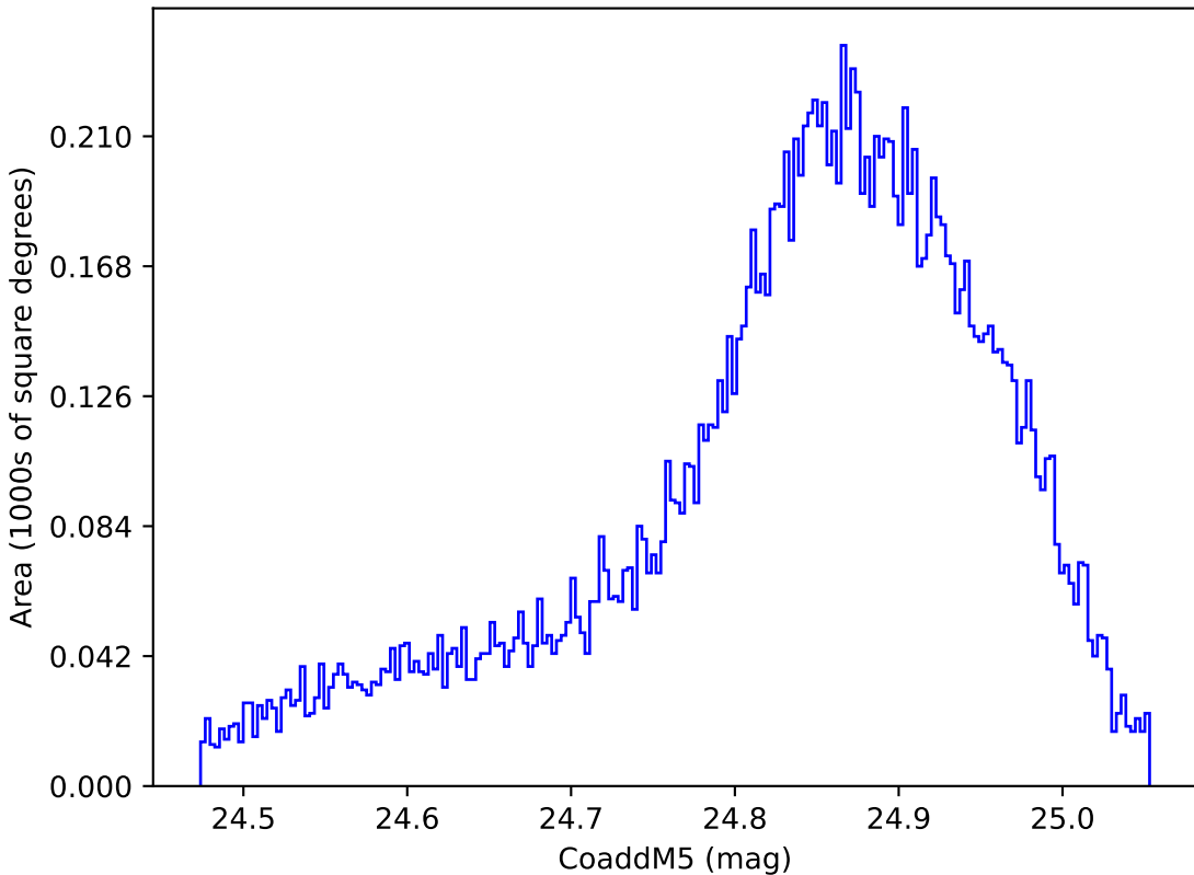
extra_ss_neo3_v3.4_10yrs WFD y band: CoaddM5
