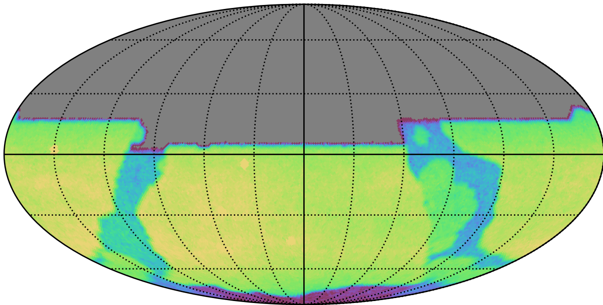
extra_ss_neo3_v3.4_10yrs All sky y band: CoaddM5
