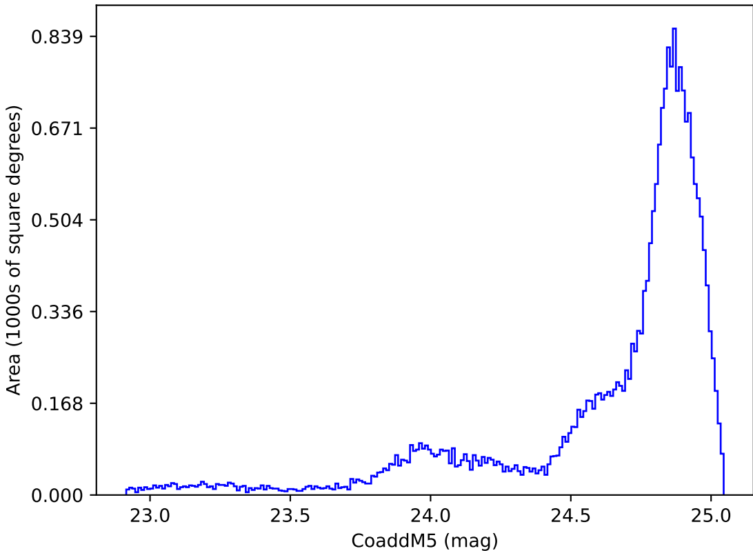
extra_ss_neo3_v3.4_10yrs All sky y band: CoaddM5
