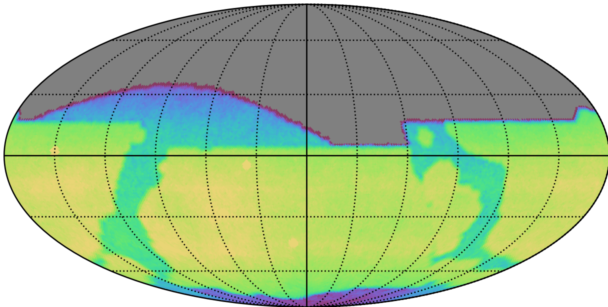
extra_ss_neo3_v3.4_10yrs All sky i band: CoaddM5
